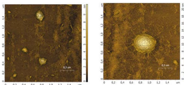
Рисунок 7 - Рельеф поверхности пленки при исследовании геля альгината натрия с добавлением \text{AgNO}_3 , \text{Na}_2\text{CO}_3 и папаина. Размер изображения 1,5x1,5 мкм
