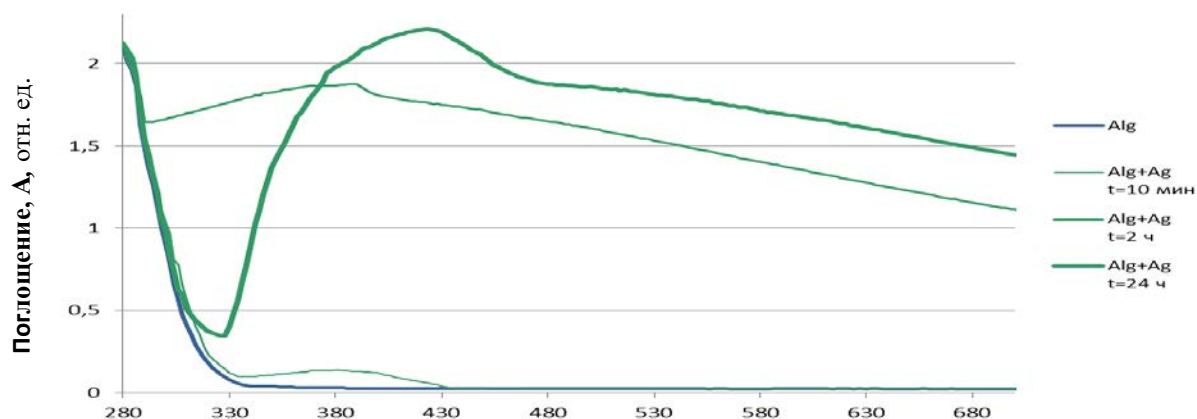
Рисунок 9 – Изменения спектров поглощения растворов альгината натрия (pH 7,5) и композиции АН+AgNO 3 при варьировании продолжительности выдержки после приготовления
